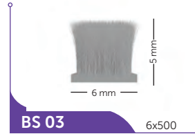
BS 03 6x500 Paket Tipi 375 m/rulo Package Type 375 m/roll Щетка 6x5 мм
